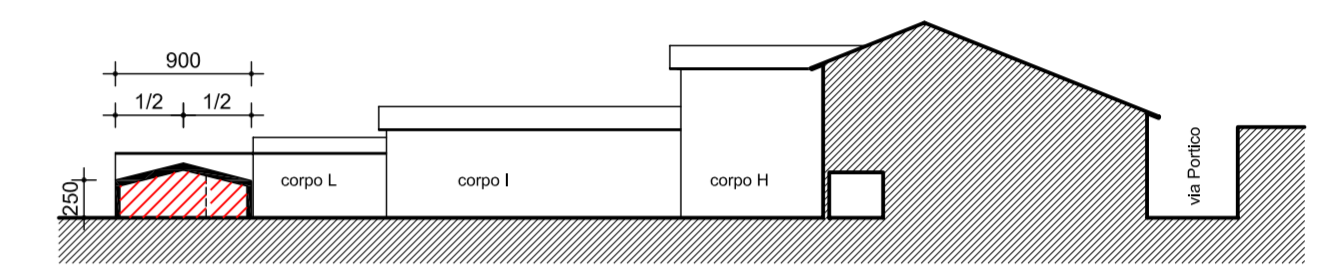
PORTICO - sez. A-A
